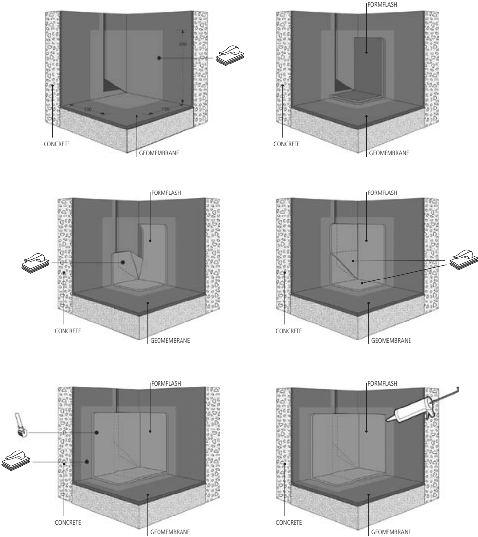
Fig. 25 : Inside corner
